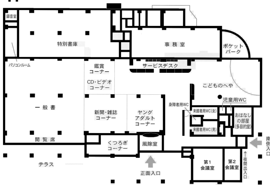
施設配置平面図
