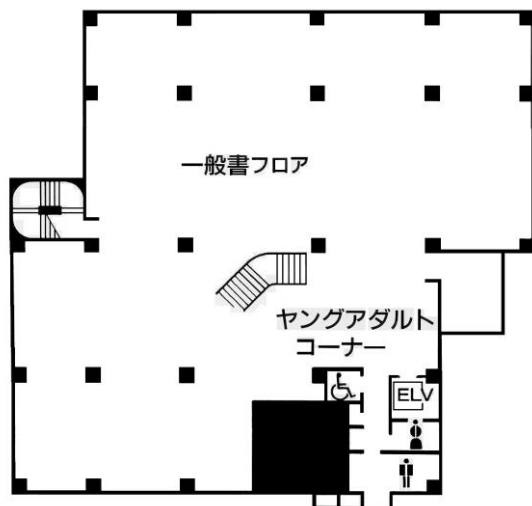
施設配置平面図
